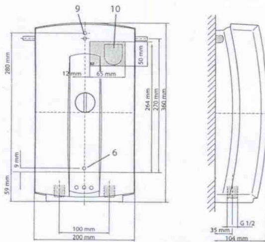
Расположение прибора
