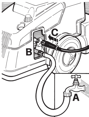
Conexión hídrica.
