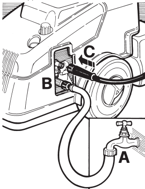
Подключение воды.
