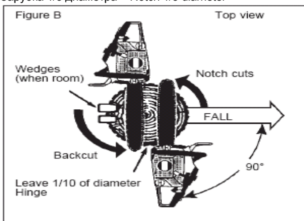
Схема В = Figure B; Вид сверху = Top view Клинья (когда пространство позволяет) =Wedges (when room) Зарубки =Notch cuts; НАПРАВЛЕНИЕ ПАДЕНИЯ = FALL; Валочный распил = Backcut; Оставьте 1/10 диаметра Leave 1/10 of diameter; Штырь=Hinge
