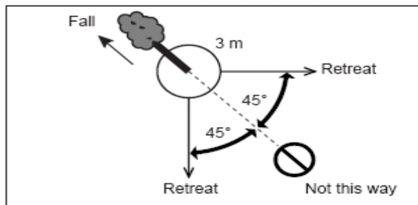
Направление падения = Fall; Отход = Retreat; Не сюда= Not this way
