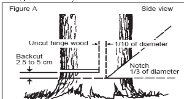
Схема А=Figure A; Вид сбоку=Side view; Оставленный штырь 1/10 диаметра = Uncut hinge wood Валочный распил от 2,5 до 5 см. = Backcut Зарубка 1/3 диаметра = Notch 1/3 diameter
