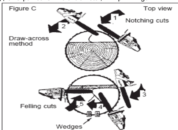
Схема С = Figure C; Вид сверху = Top view; Пропилы зарубки = Notching cuts; Метод протягивания пилы = Draw-across method; Валочные пропилы = Felling cuts; Клинья=Wedges
