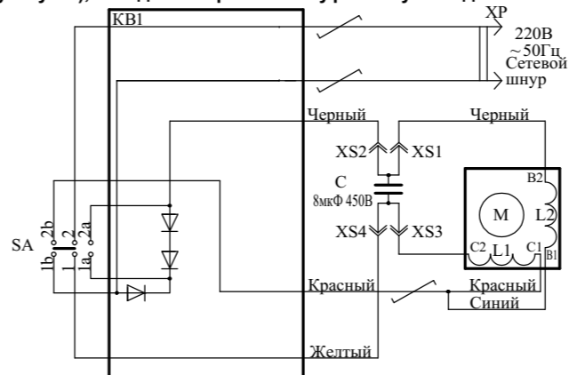
Рисунок 2 - Схема электрическая принципиальная
