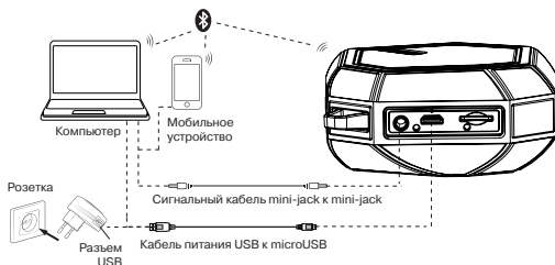
Рис. 2. Схема подключения
