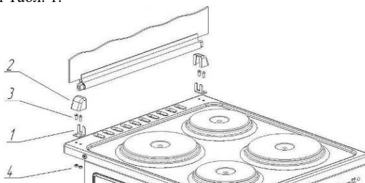
Рис. 6. Установка стеклянной крышки стола.
