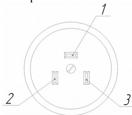
Рис. 1. Подключение розетки
