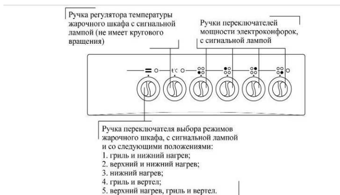
Рис. 8. Передняя панель плиты СТЕ-54 sWh
