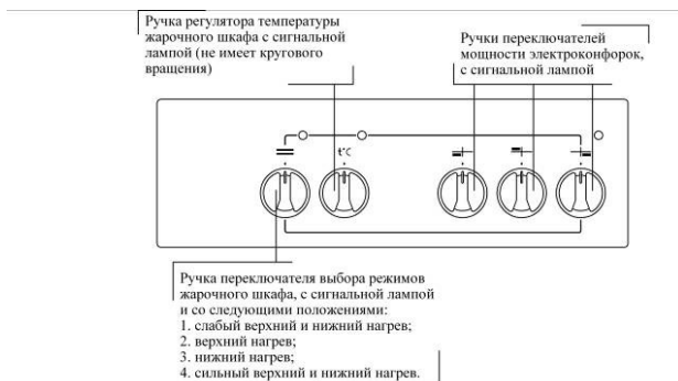
Рис. 7. Передняя панель плиты СТЕ-53 Wh
