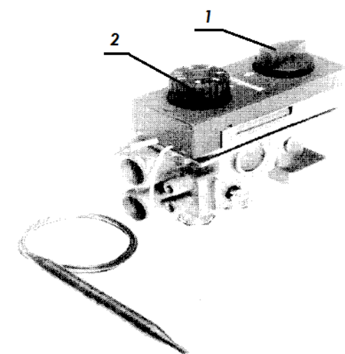
Комбинированный газовый клапан V5475
