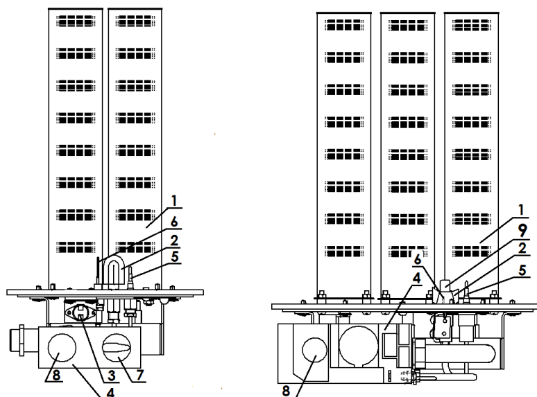
Рис. 12 Горелки УГч-19, УГч-29 к котлам КЧ-Г-16, КЧ-Г-25.
