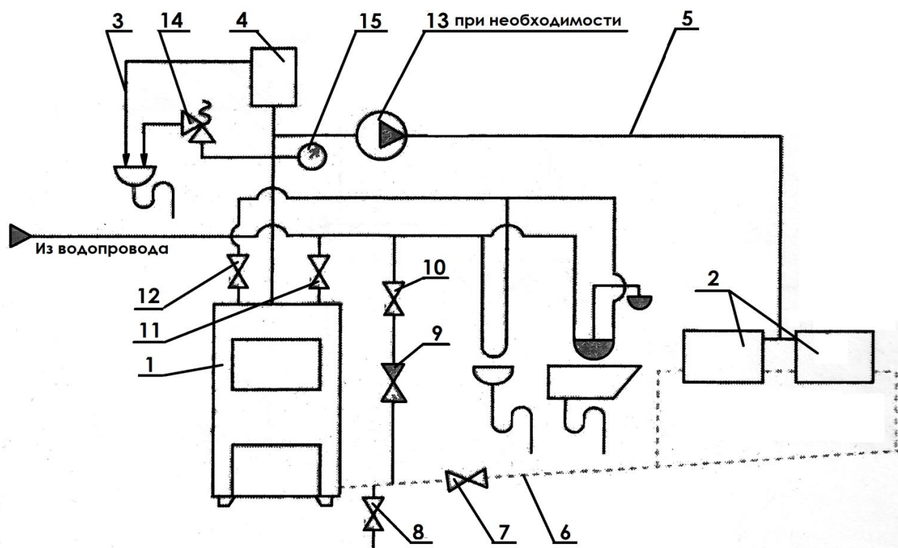
Открытая система отопления
