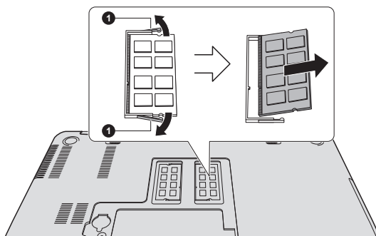
Рисунок 4-14 Удаление модуля памяти
