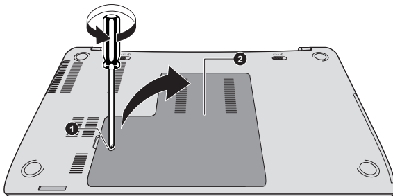
Рисунок 4-11 Снятие крышки отсека модулей памяти
