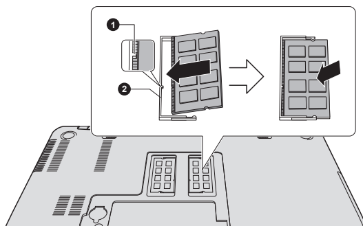
Рисунок 4-12 Установка модуля памяти
