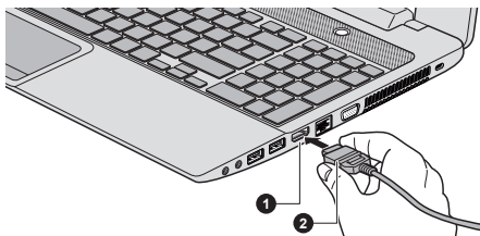
Рисунок 4-18 Подключение к порту выхода HDMI
