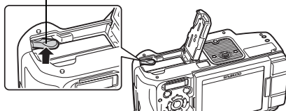
Защелка аккумулятора
